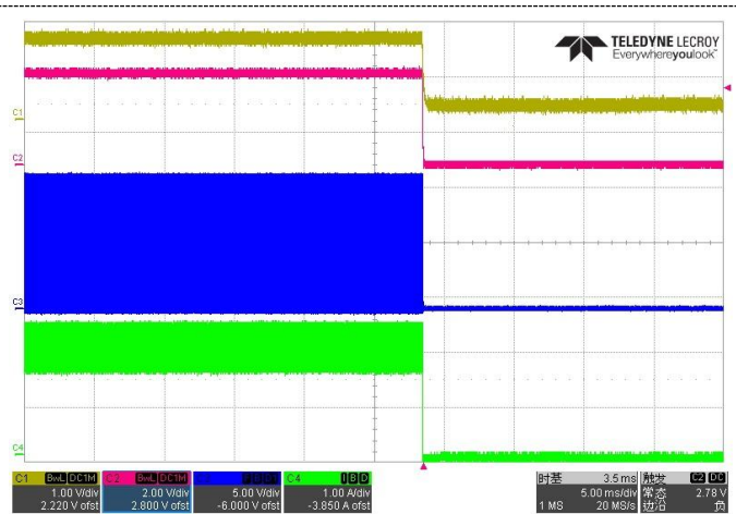
Iout=2A
