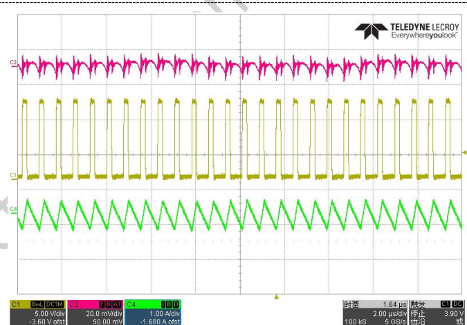
Iout=0A
