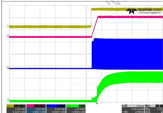
Iout=2A
